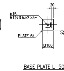
BASE PLATE L-50
